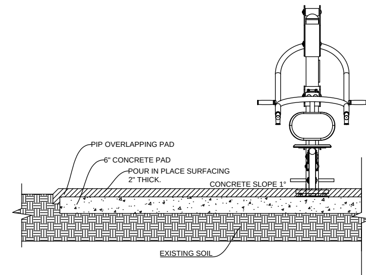
PIP Wrap-Around
